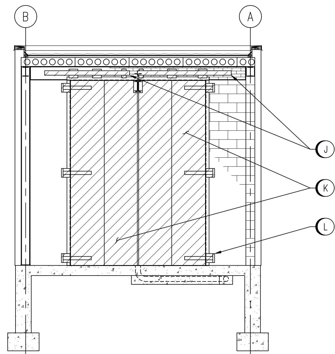
SECTION SCALE: 1 : 50
